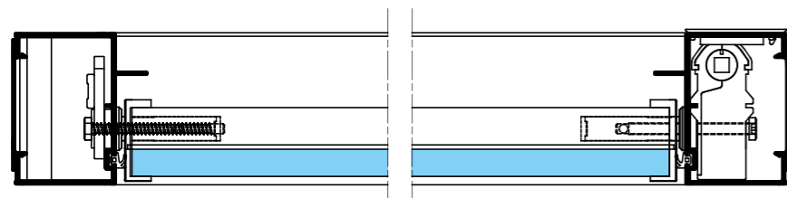
Coupe horizontale
