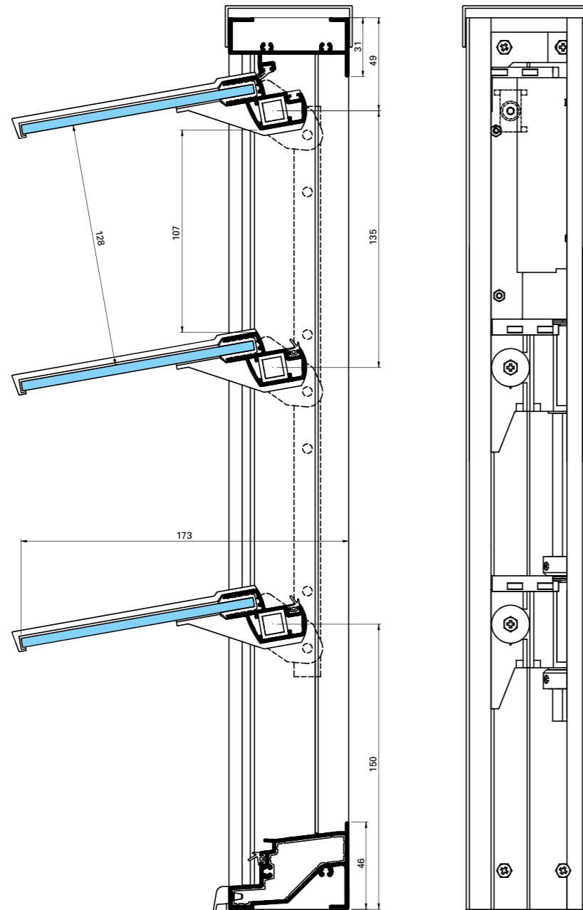
Coupes verticales
